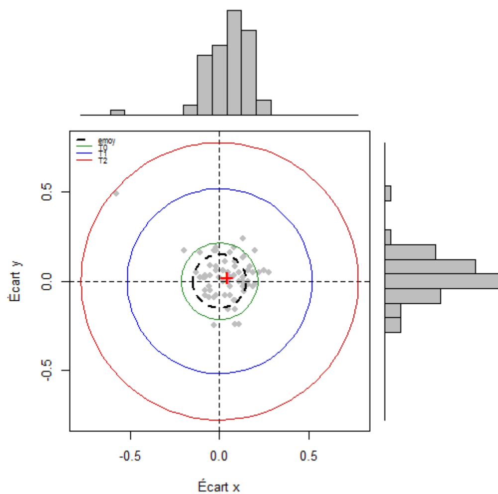
Représentation graphique des écarts planimétriques effectuée avec le logiciel R
