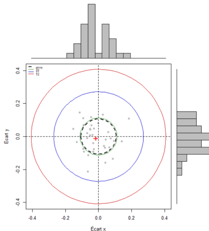
Représentation graphique des écarts planimétriques effectuée avec le logiciel R
